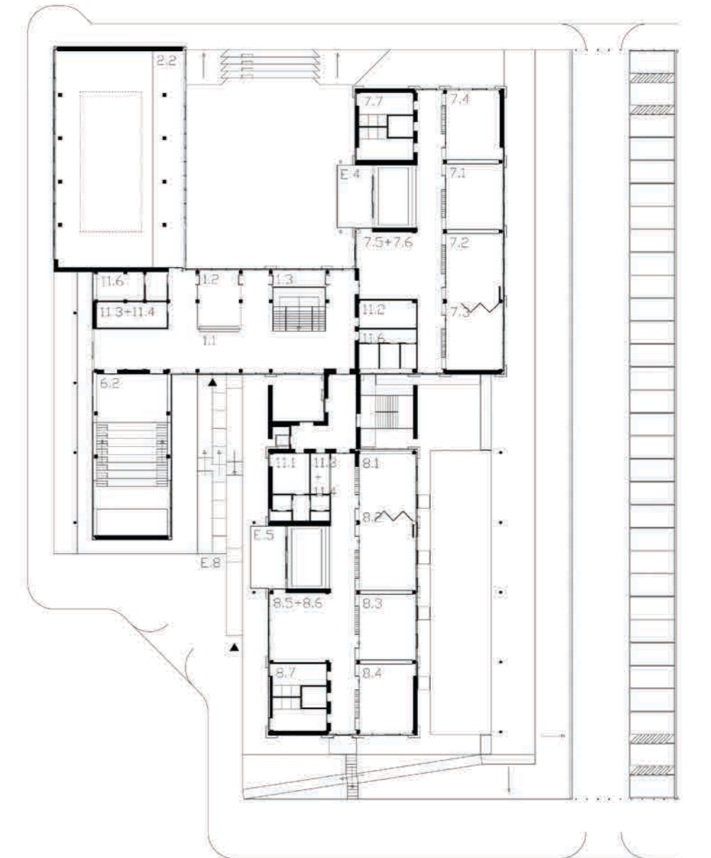
PLANIMETRIA PIANO RIALZATO
