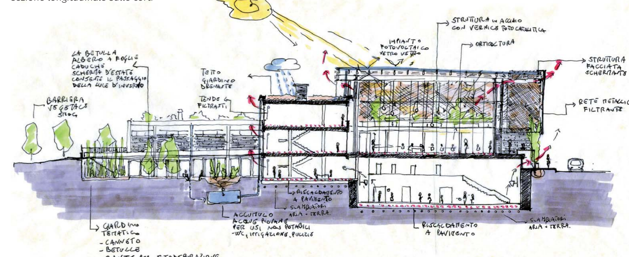
sezione longitudinale sulle corti
